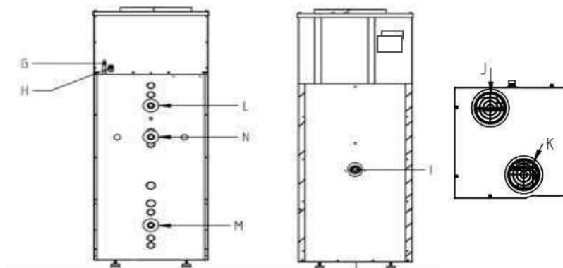
Illustration : Anslutningar och komponenter (baksida, sida och upptill)
