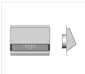
art.nr: 20654 Väggdon VDP120 för reg/våtluft
